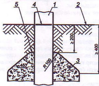
1 — опора; 2 — поверхность покрытия игровой площадки; 3 — фундамент; 4 — базовая отметка заглибления; 5 — верх фундамента
