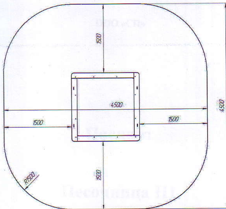
Рис.3 Зона безопасности
